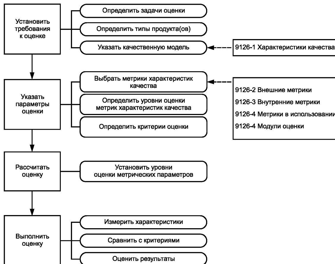
Рисунок D.1 — Диаграмма согласно ГОСТ Р ИСО/МЭК 25040 [8]
